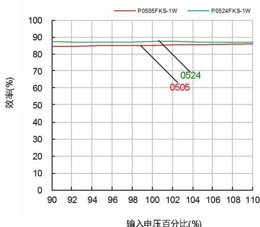
效率与输入电压关系曲线图(满载)
