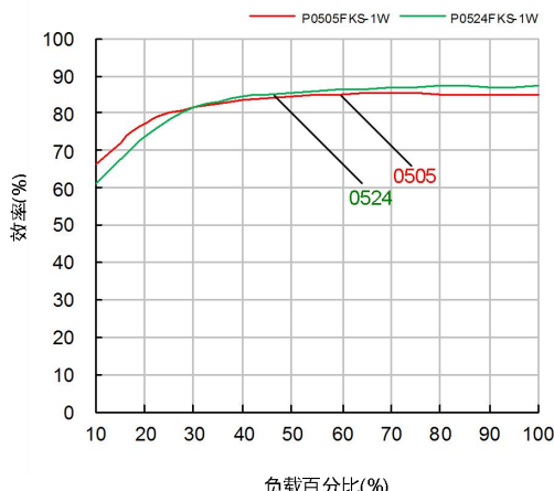
效率与负载关系曲线图(标称输入电压)
