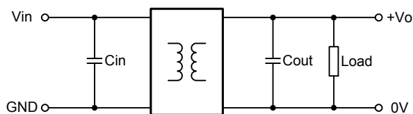
图 1 应用电路图
